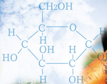
ブドウ糖 (C 6 H 12 O 6 )
