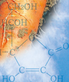
ビタミンC (C 6 H 8 O 6 )
