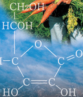
ビタミンC (C 6 H 8 O 6 )
