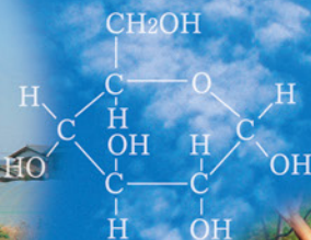
ブドウ糖 (C 6 H 12 O 6 )
